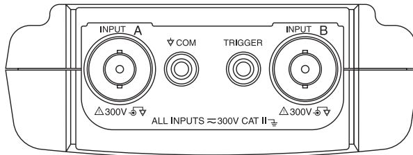
Figur 6. Måletilkoblinger
