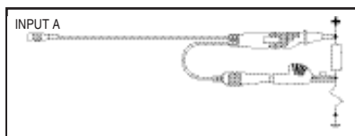
(Riktig jording) Skjermen på testledningen er tilkoblet jord.
