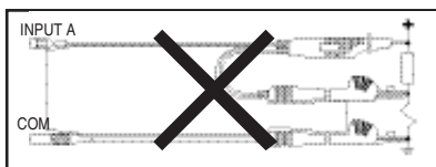
(Feil jording) Jordingsløfe ved dobbel jording på forskjellig jord.
